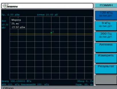
Рис. 8. Отклик квазипикового детектора на радиоимпульс 300 МГц с частотой повторения 100 Гц и длительностью 1 мкс
