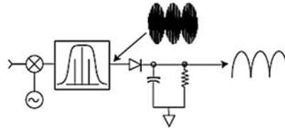
Рис. 1. Пиковый детектор
