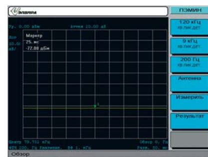
Рис. 12. Отклик квазипикового детектора 200 Гц на видеоимпульс с частотой повторения 25 Гц и длительностью 850 нс
