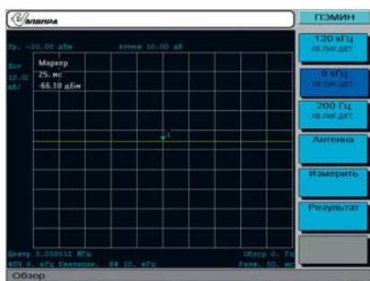
Рис. 10. Отклик квазипикового детектора 9 кГц на видеоимпульс с частотой повторения 100 Гц и длительностью 15 нс
