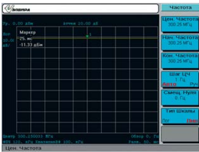
Рис. 7. Отклик квазипикового детектора на радиоимпульс 300 МГц с частотой повторения 250 кГц и длительностью 1 мкс
