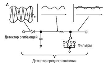
Рис. 2. Детектор средних значений
