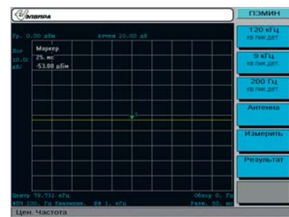
Рис. 11. Отклик квазипикового детектора 200 Гц на видеоимпульс с частотой повторения 1 кГц и длительностью 850 нс
