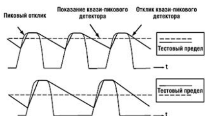
Рис. 3. Принцип работы квазипикового детектора
