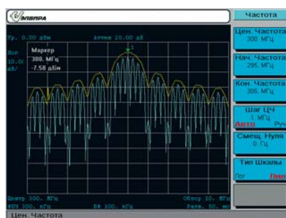
Рис. 5. Радиоимпульс 300 МГц с частотой повторения 250 кГц и длительностью 1 мкс на экране СК4-БЕЛАН 32
