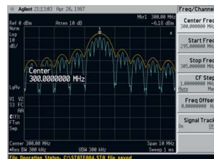
Рис. 6. Радиоимпульс 300 МГц с частотой повторения 250 кГц и длительностью 1 мкс на экране Agilent E4440A
