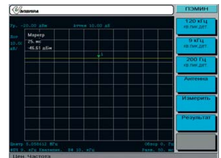
Рис. 9. Отклик квазипикового детектора 9 кГц на видеоимпульс с частотой повторения 50 кГц и длительностью 15 нс
